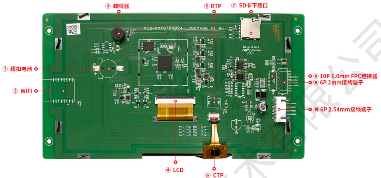
端口定义
